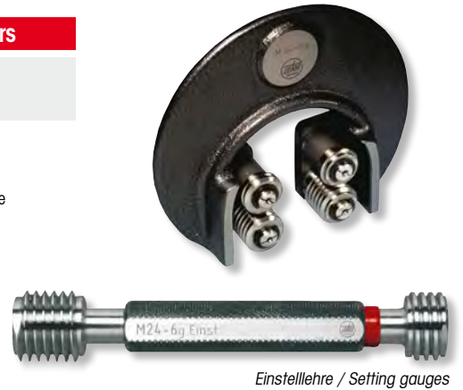
Einstelllehre / Setting gauges
